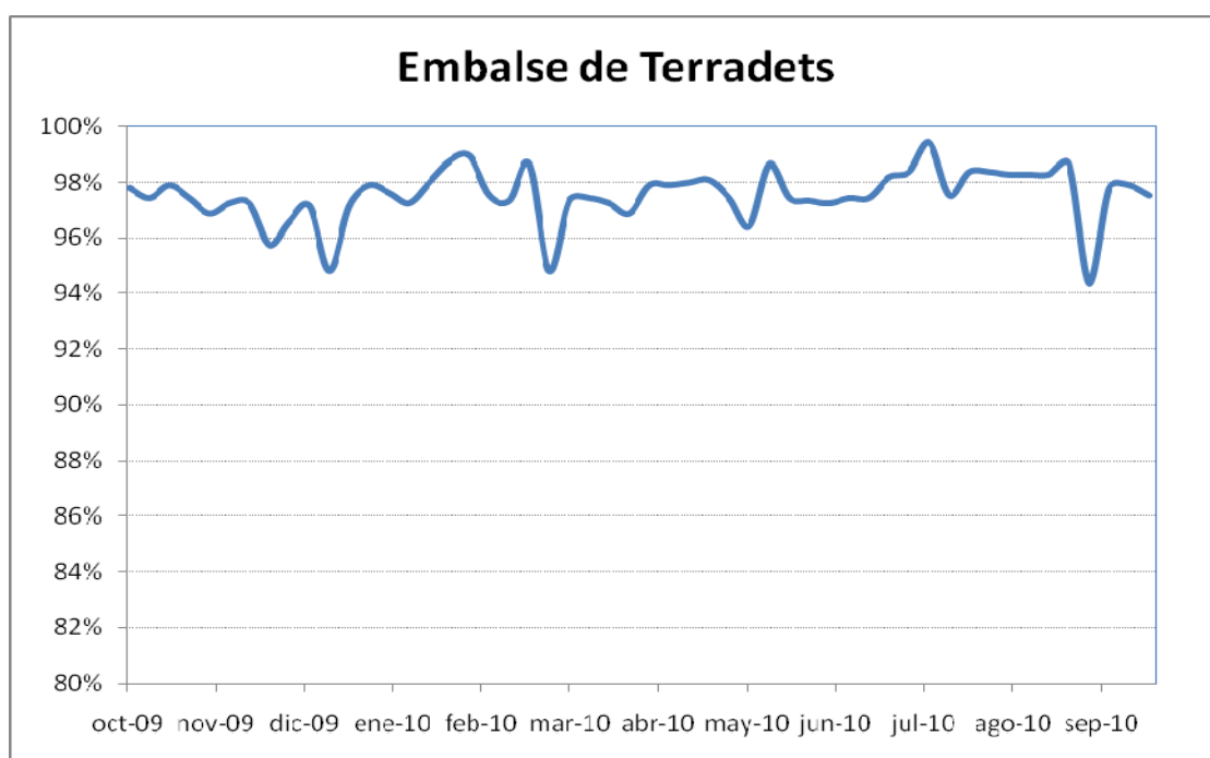
GRÁFICO 1 VOLUMEN EMBALSADO (%) DURANTE EL AÑO HIDROLÓGICO 2009-2010
