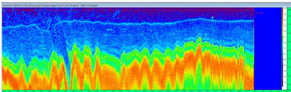
Figura 14. Ejemplo de un ecograma obtenido con el haz vertical en el embalse de Tramacastilla
