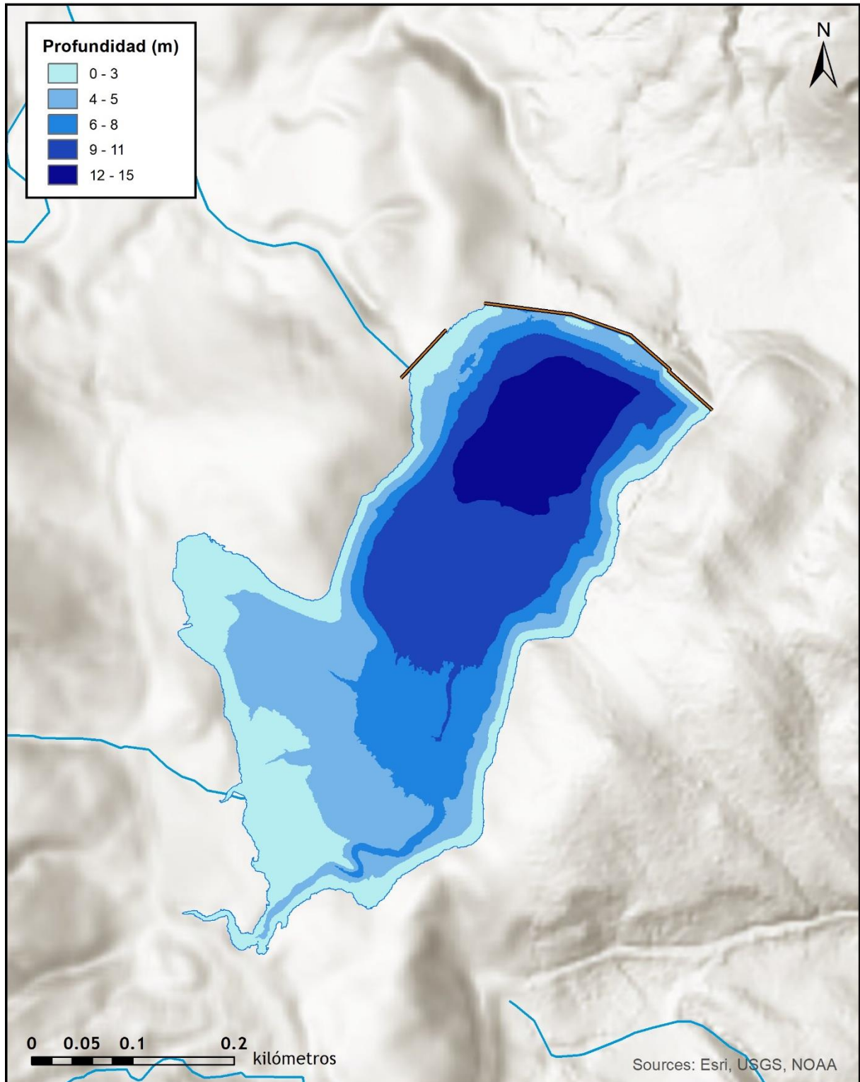
Figura 4. Batimetría del embalse de Tramacastilla
