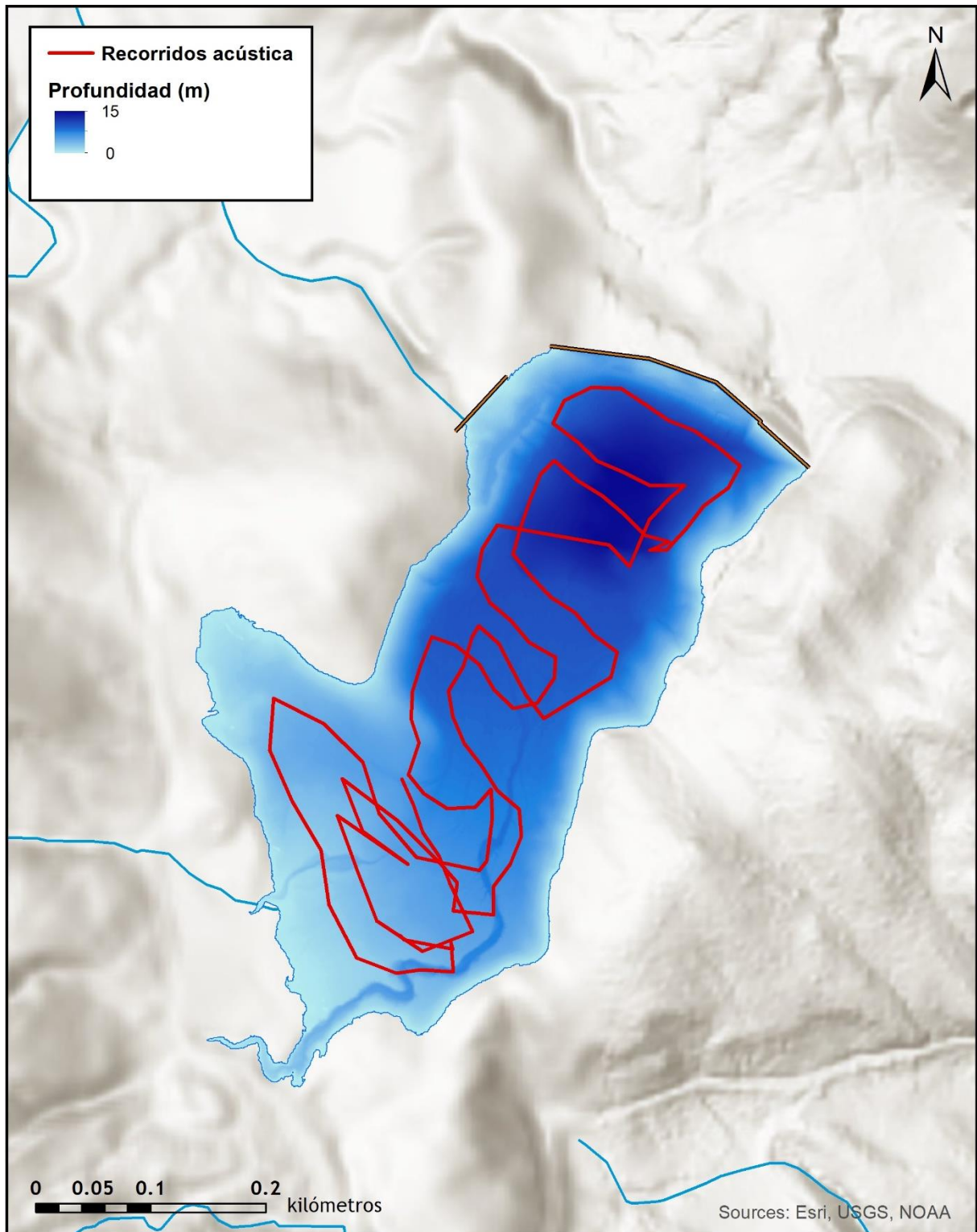
Figura 13. Recorridos del sondeo hidroacústico en el embalse de Tramacastilla
