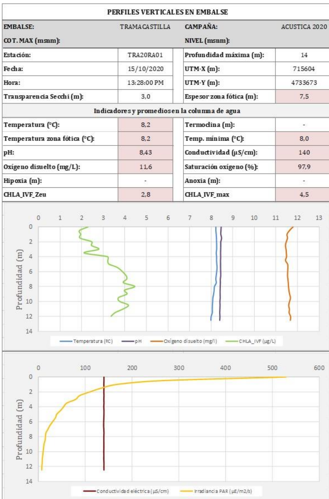
Figura 6. Perfiles físico-químicos realizados en el embalse de Tramacastilla
