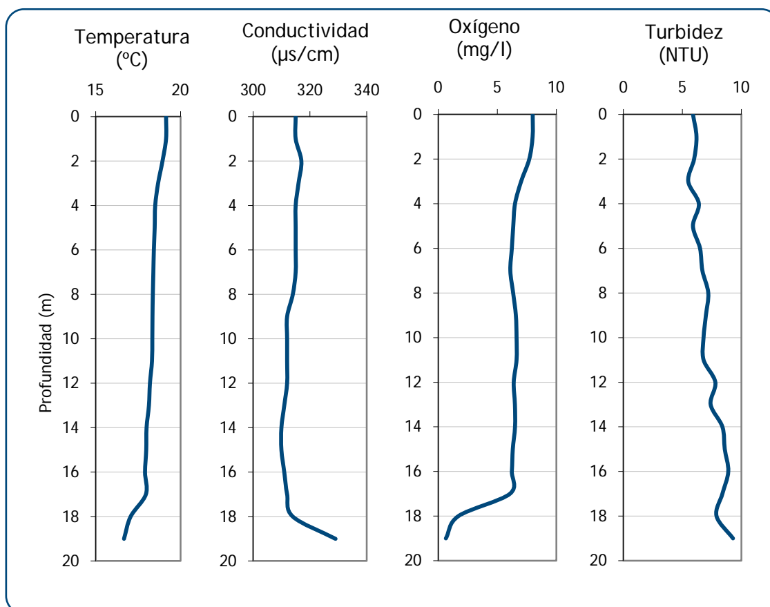
Figura 3. Perfiles de temperatura, conductividad, turbidez y oxígeno disuelto en el momento del muestreo
